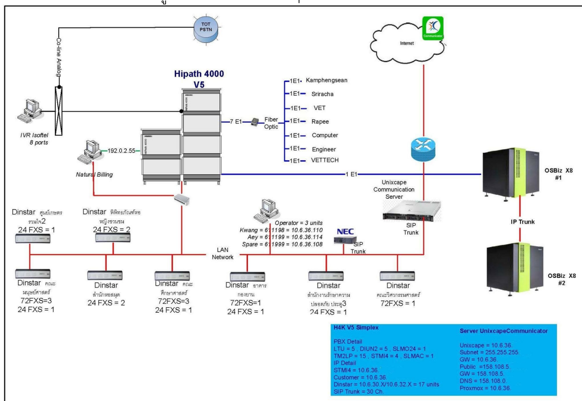
ภาพที่ ก-3-10 การปรับเปลี่ยนระบบอะนาล็อกเป็น ระบบไอพีแอดเดรส
